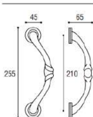
Maniglione singolo Door pull handle
